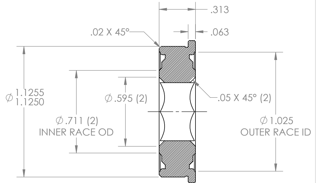
SECTION A-A
